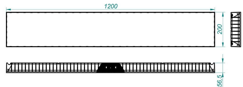
Рисунок 1б Светильник «L-school 16/Em, L-school 32/Em, L-school 55/Em»
